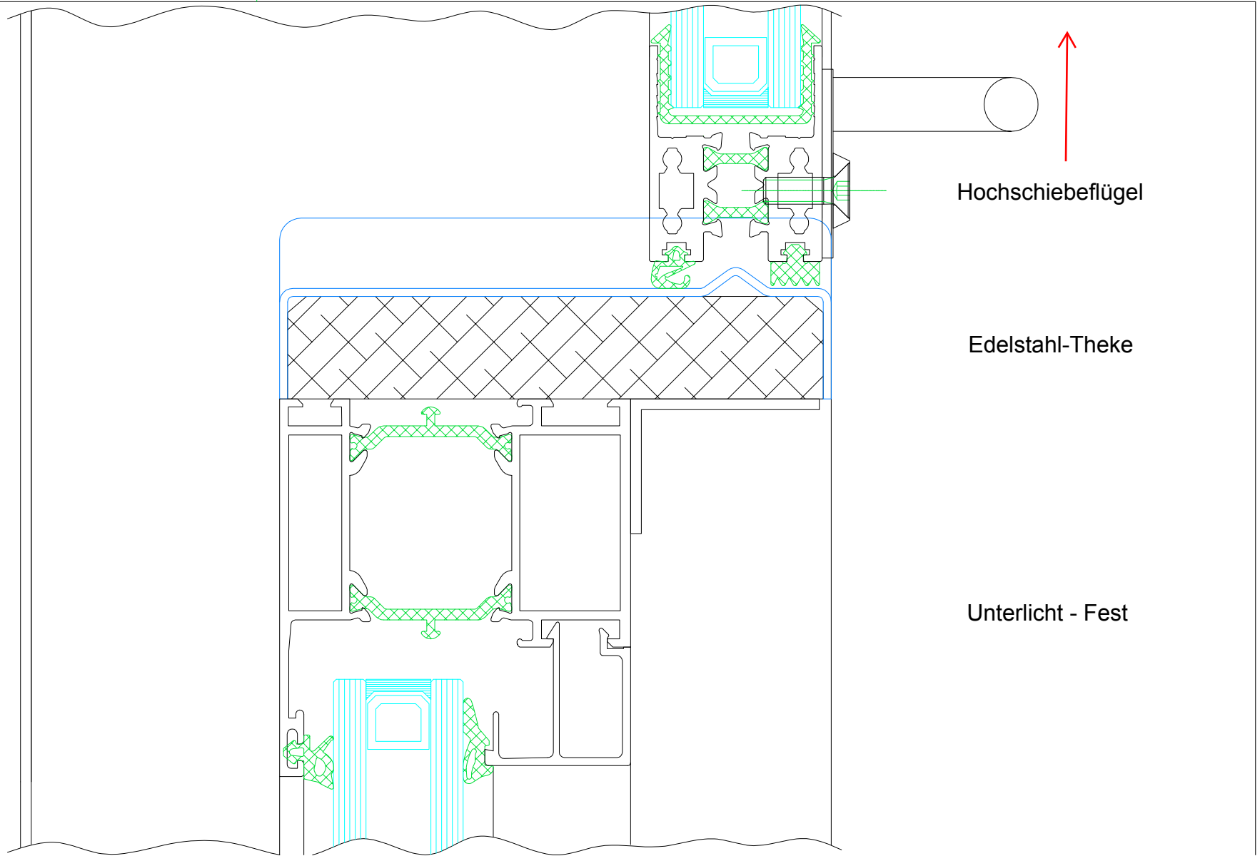
Hochschiebefenster Alu Typ B Warmprofil mit Edelstahltheke und Wassernase ( z.B. für 3teil. Verkaufsfenster)
