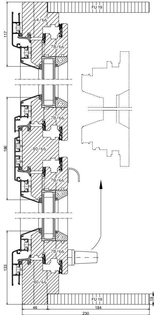
® (Holz-Metall) - Ausführung VSF-HoMe 21021 / 21041 / 21051 / 31061 / 31071 Schnitt D - D
