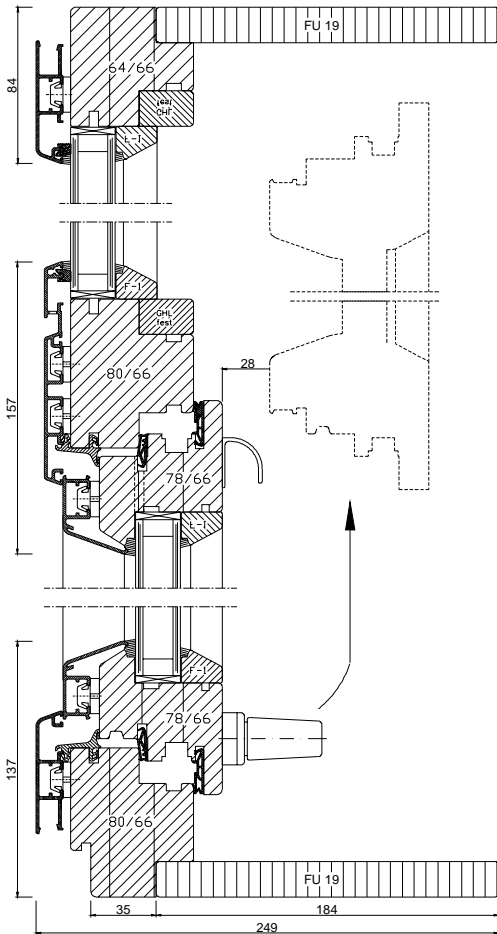
® (Holz-Metall) - Ausführung VSF-HoMe 11011 Schnitt C - C
