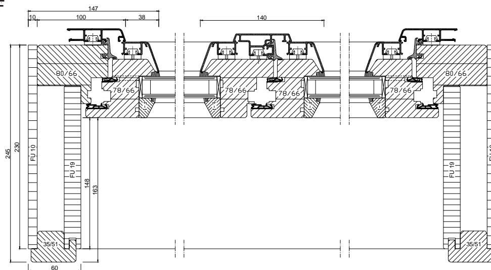
® (Holz-Metall) - Ausführung VSF-HoMe 31061 Schnitt F - F
